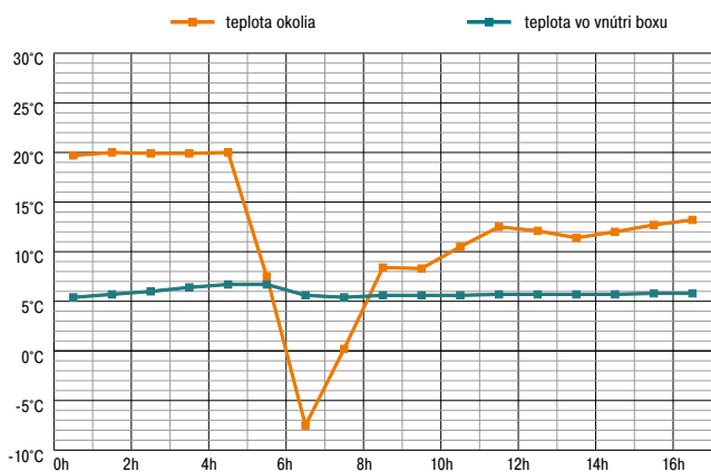
Teplotná krivka termo-izolačného setu zimná
